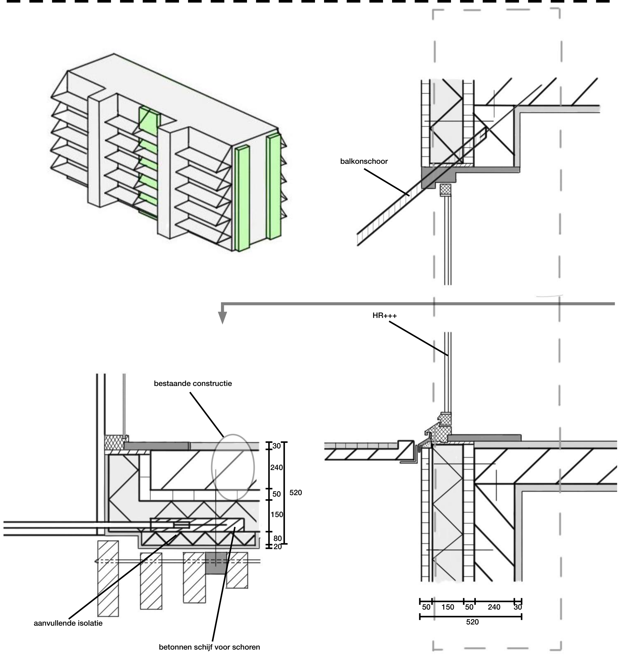
-DETAIL SCHIJVEN
